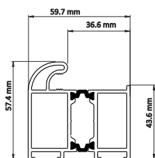
Profil ościeżnicy KMT ENERGY 60
