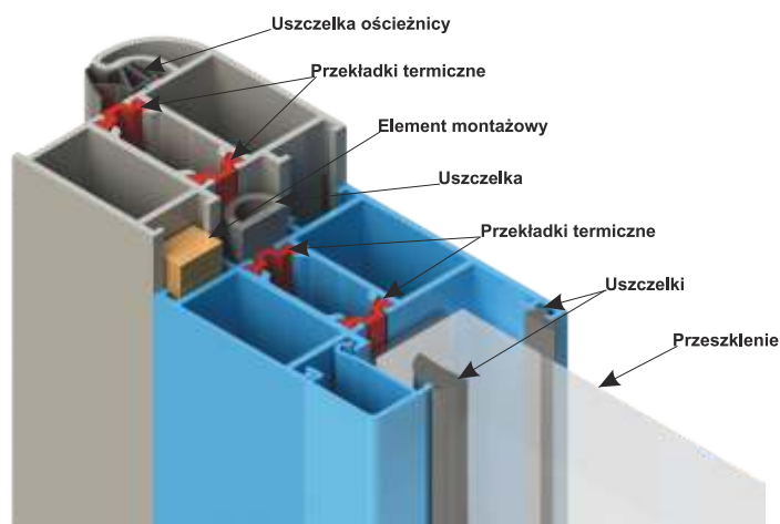
Profil ościeżnicy ENERGY 60
