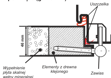
PRZEKRÓJ SKRZYDŁA - P.poż. EI 30 (gr. 46 mm)
