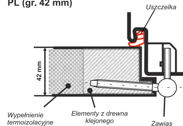
PRZEKRÓJ SKRZYDŁA - PL (gr. 42 mm)
